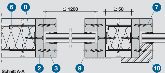
Schnitt A-A
