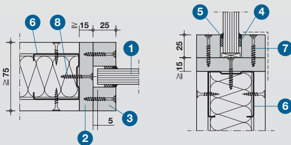
Detail B - Wandanschluss
